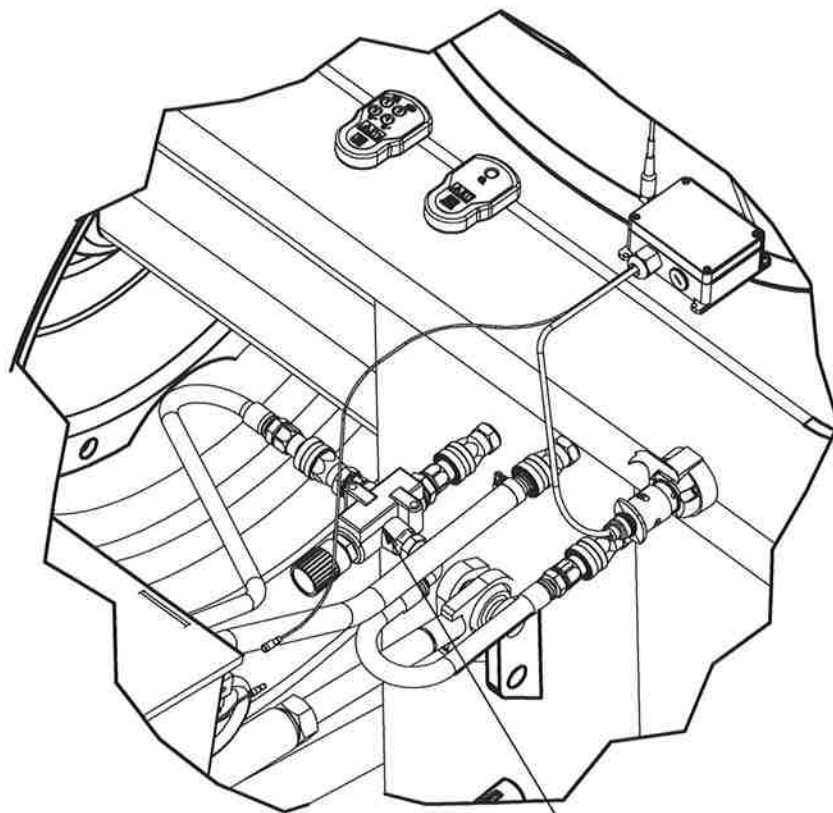
Oljemengdereguleringsventil
