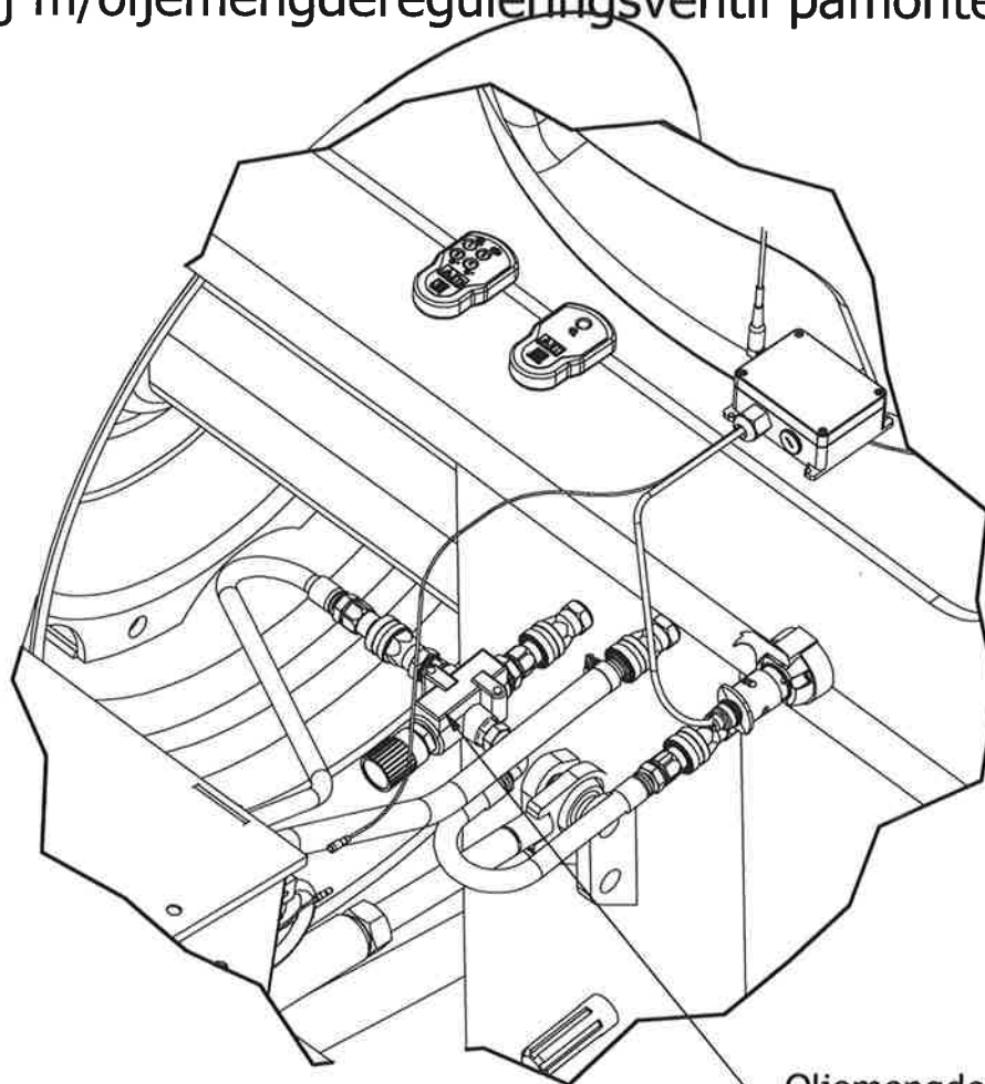
Oljemengdereguleringsventil
